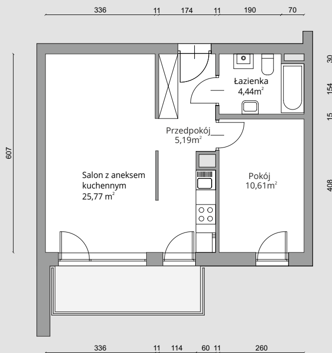
RZUT KONDYGNACJI
