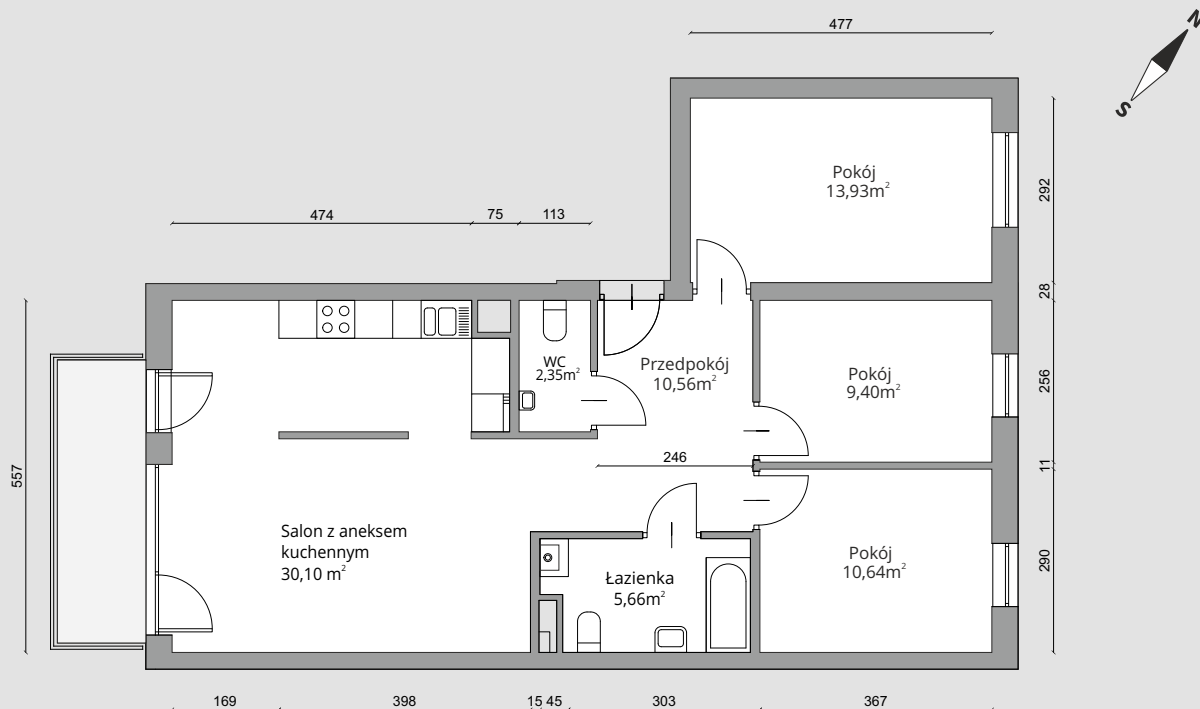
RZUT KONDYGNACJI
