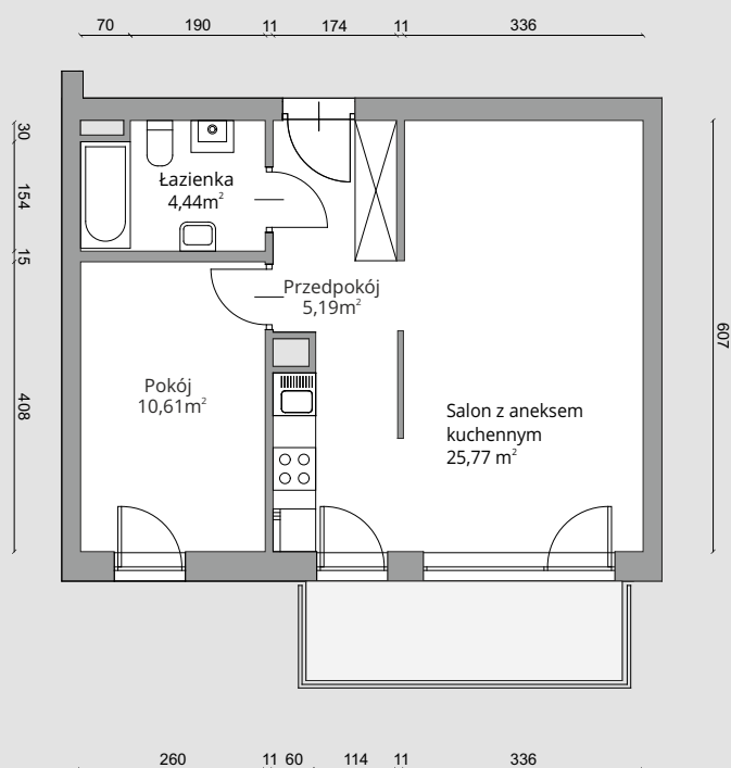
RZUT KONDYGNACJI
