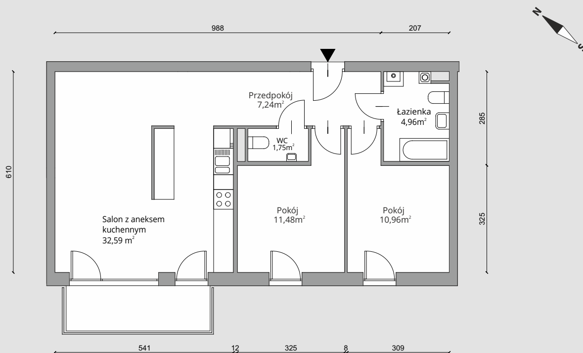
RZUT KONDYGNACJI
