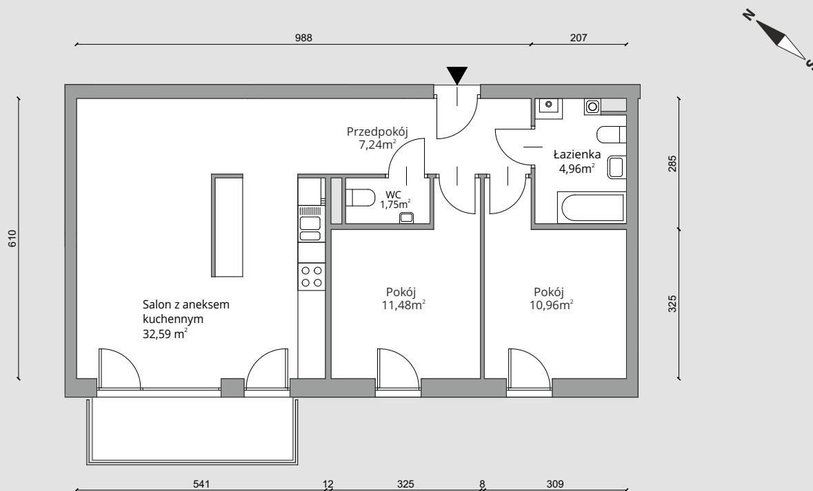
RZUT KONDYGNACJI
